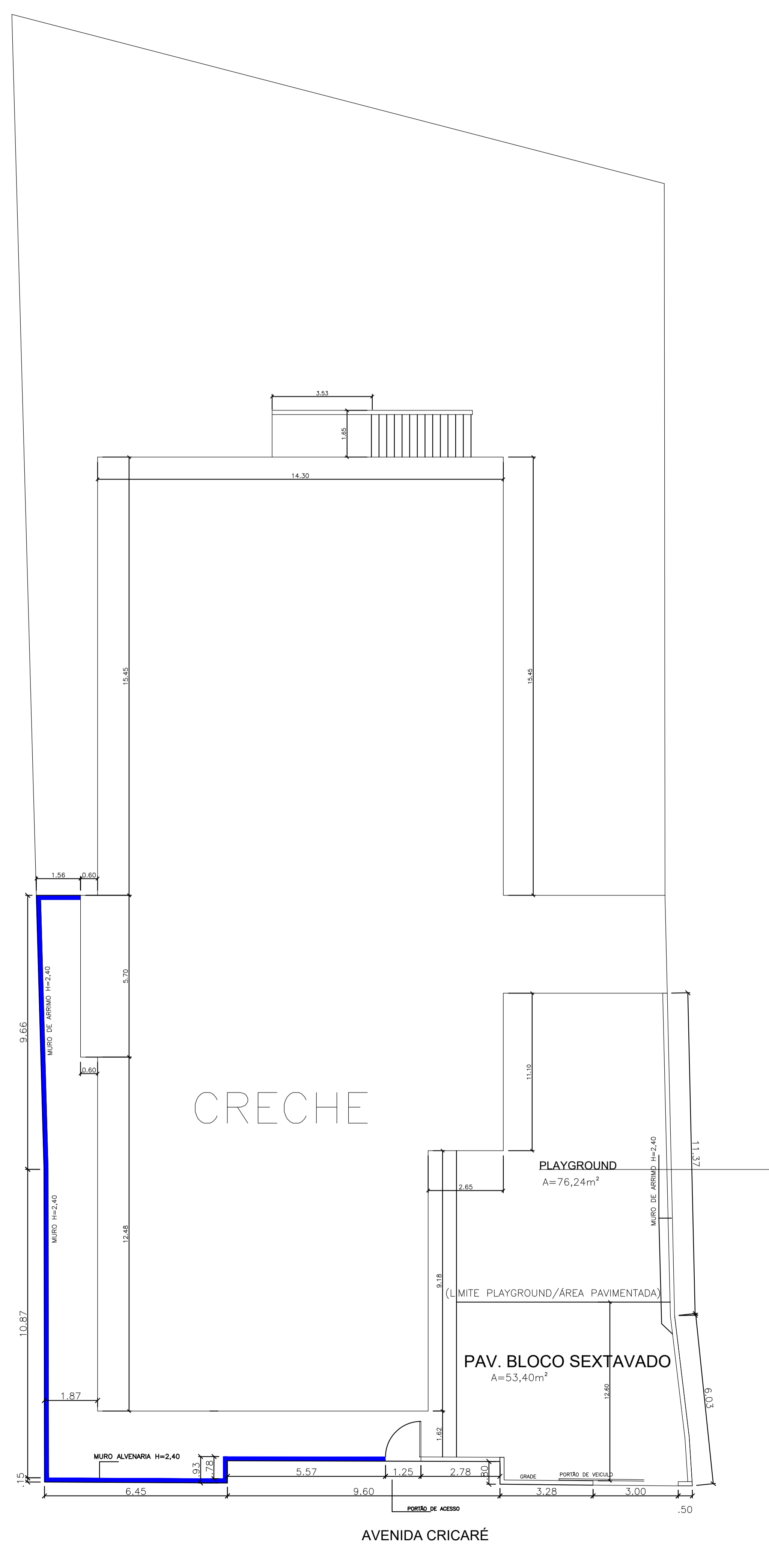
PLANTA DE CONSTRUÇÃO ESC. - 1/50
