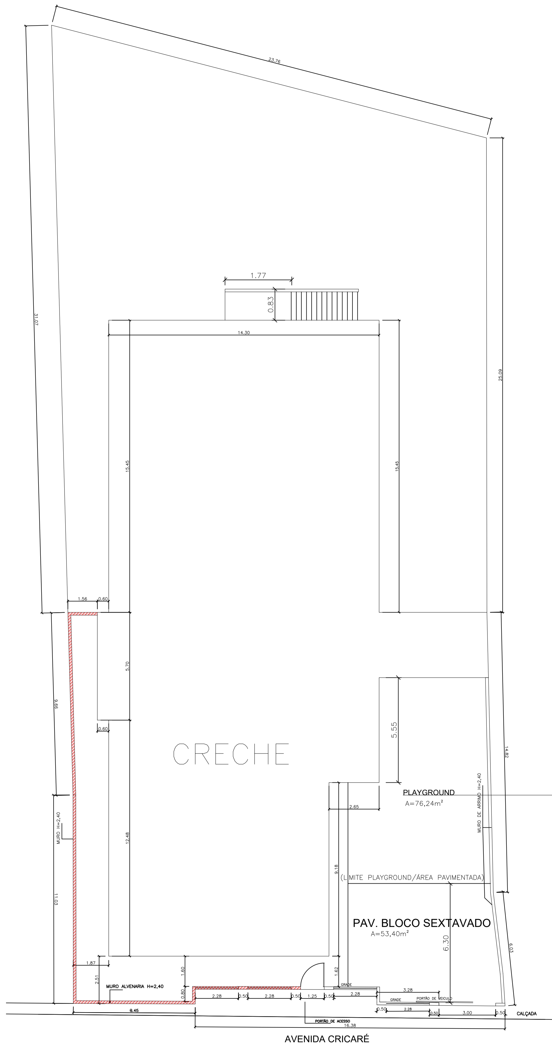
PLANTA DE DEMOLIÇÃO ESC. - 1/50
