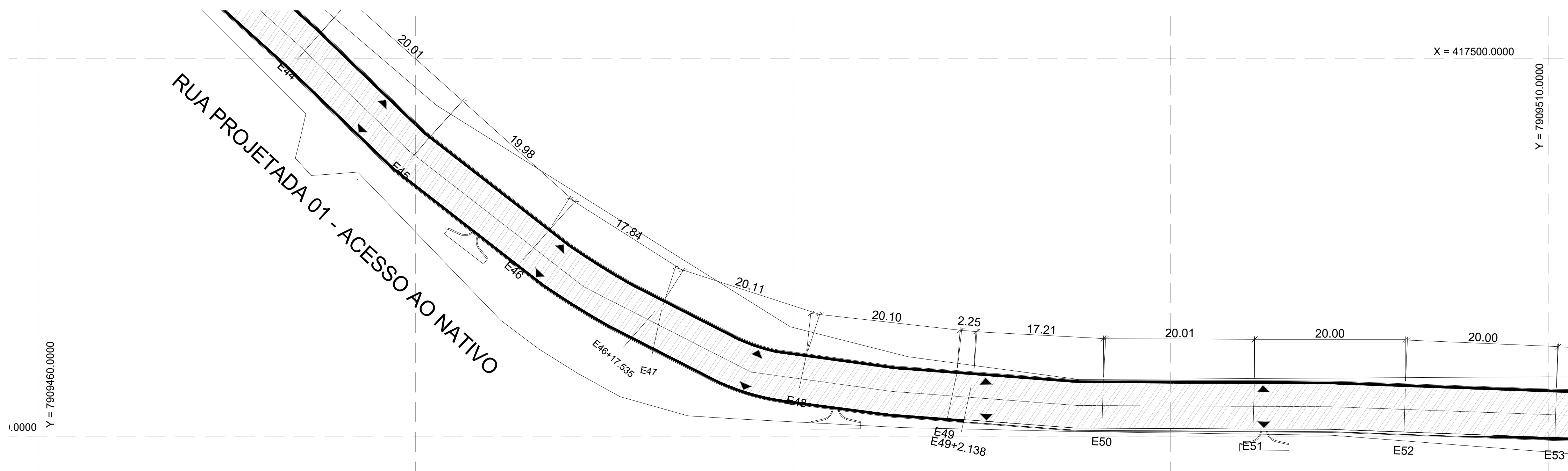
PLANTA BAIXA - PAVIMENTAÇÃO 05 TRECHO 05 esc 1:350
