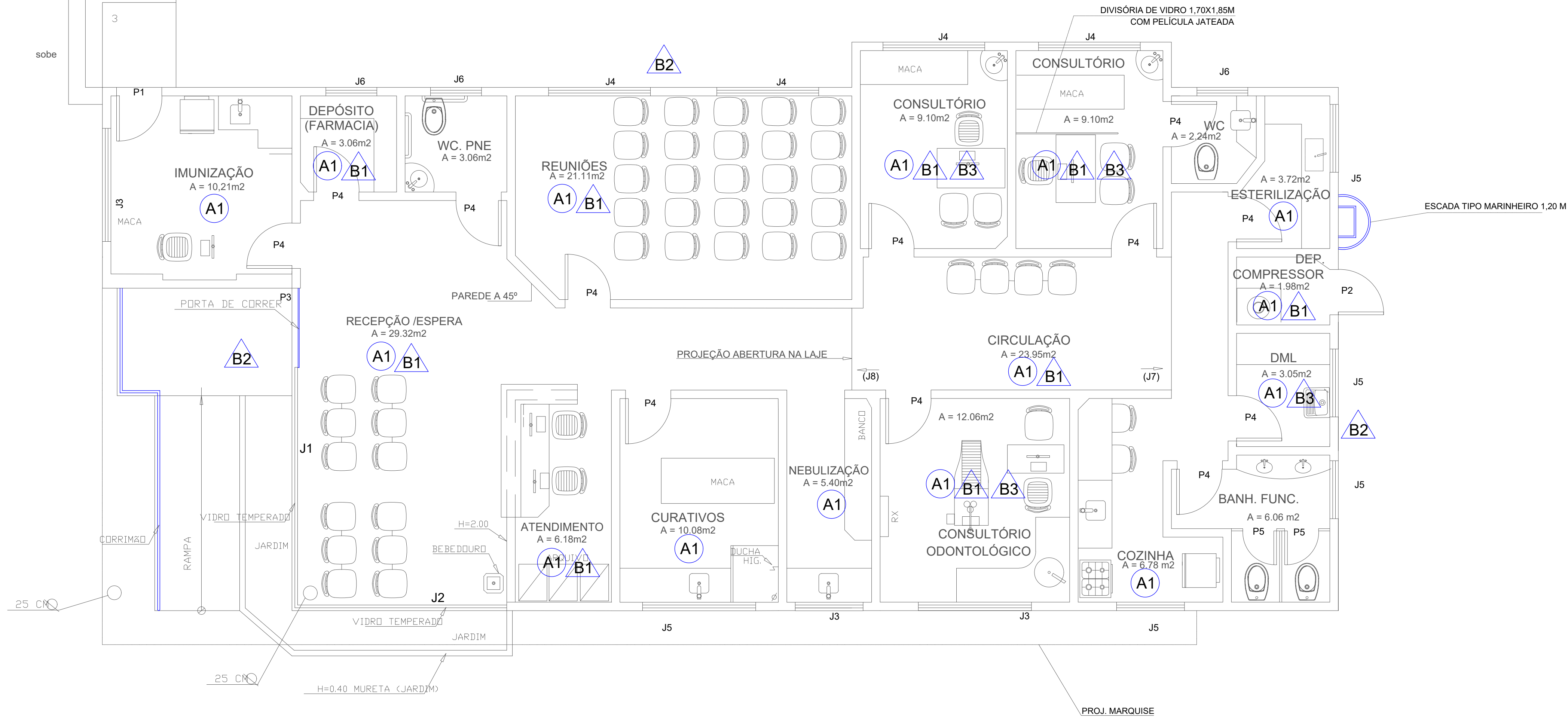
PLANTA BAIXA DE REFORMA ESC. 1/50 ÁREA: 186.17m²
