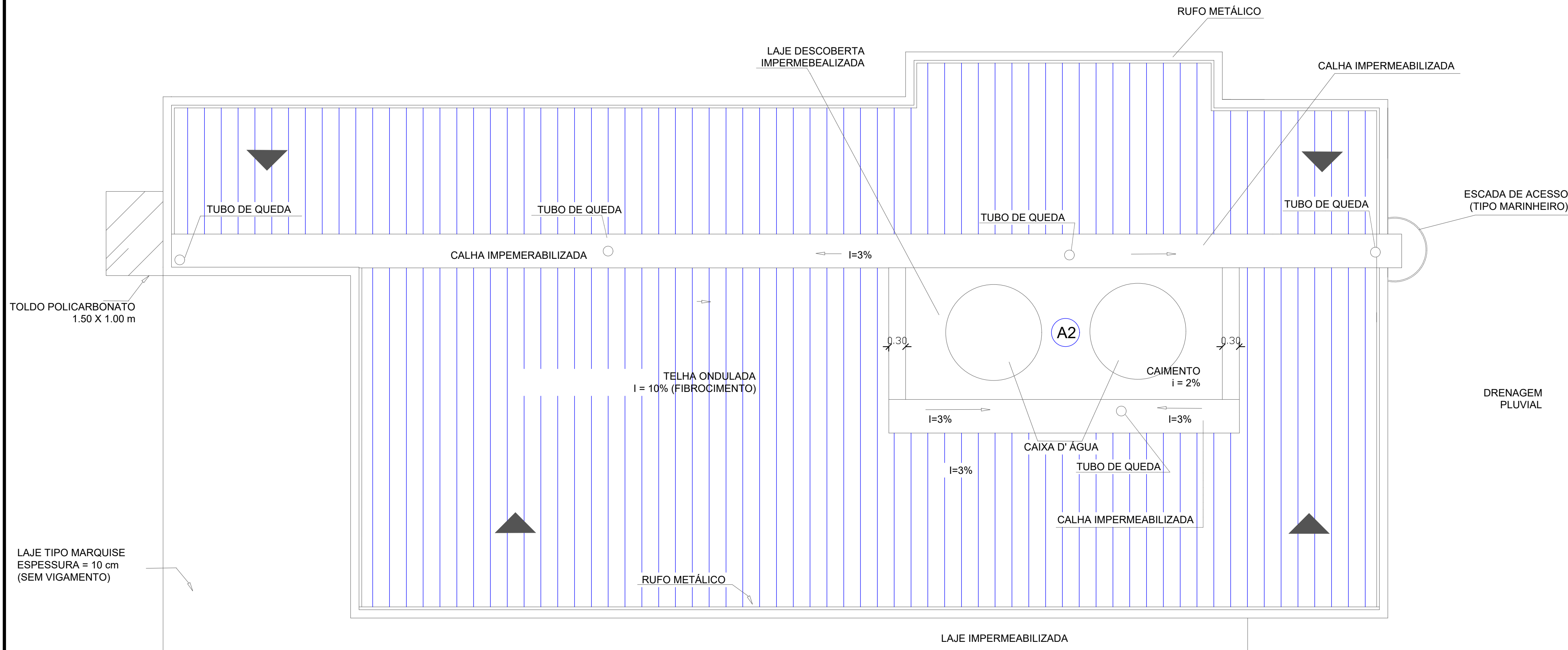
PLANTA BAIXA DE REFORMA ESC. 1/50 ÁREA: 186.17m²
