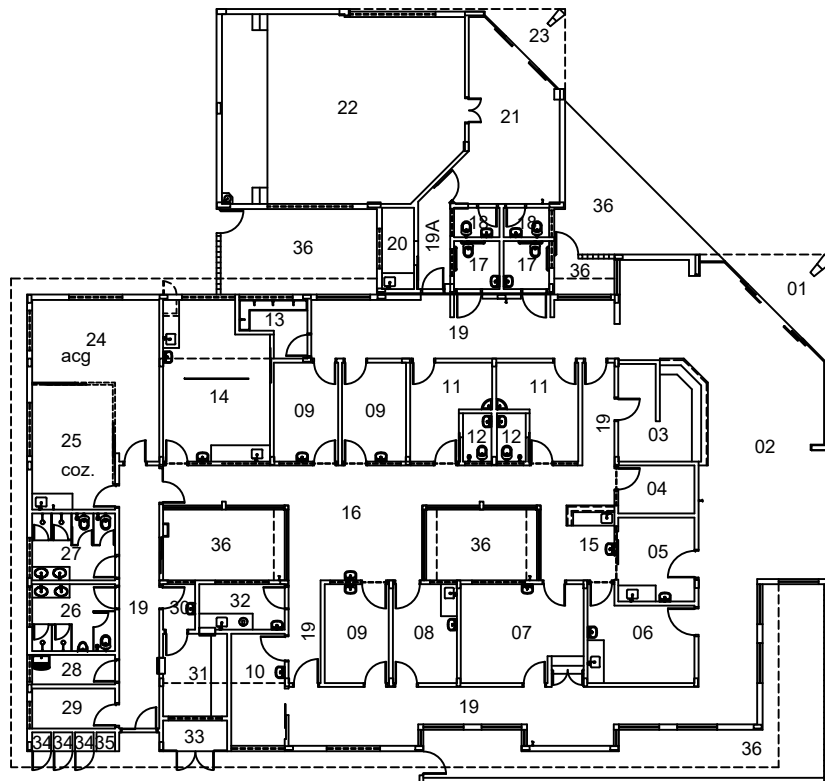
1 LEVANTAMENTO 1/100
