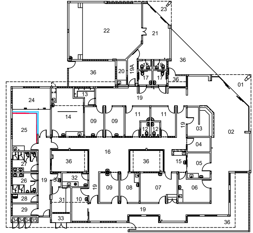
1 PLANTA DE REFORMA 1/200
