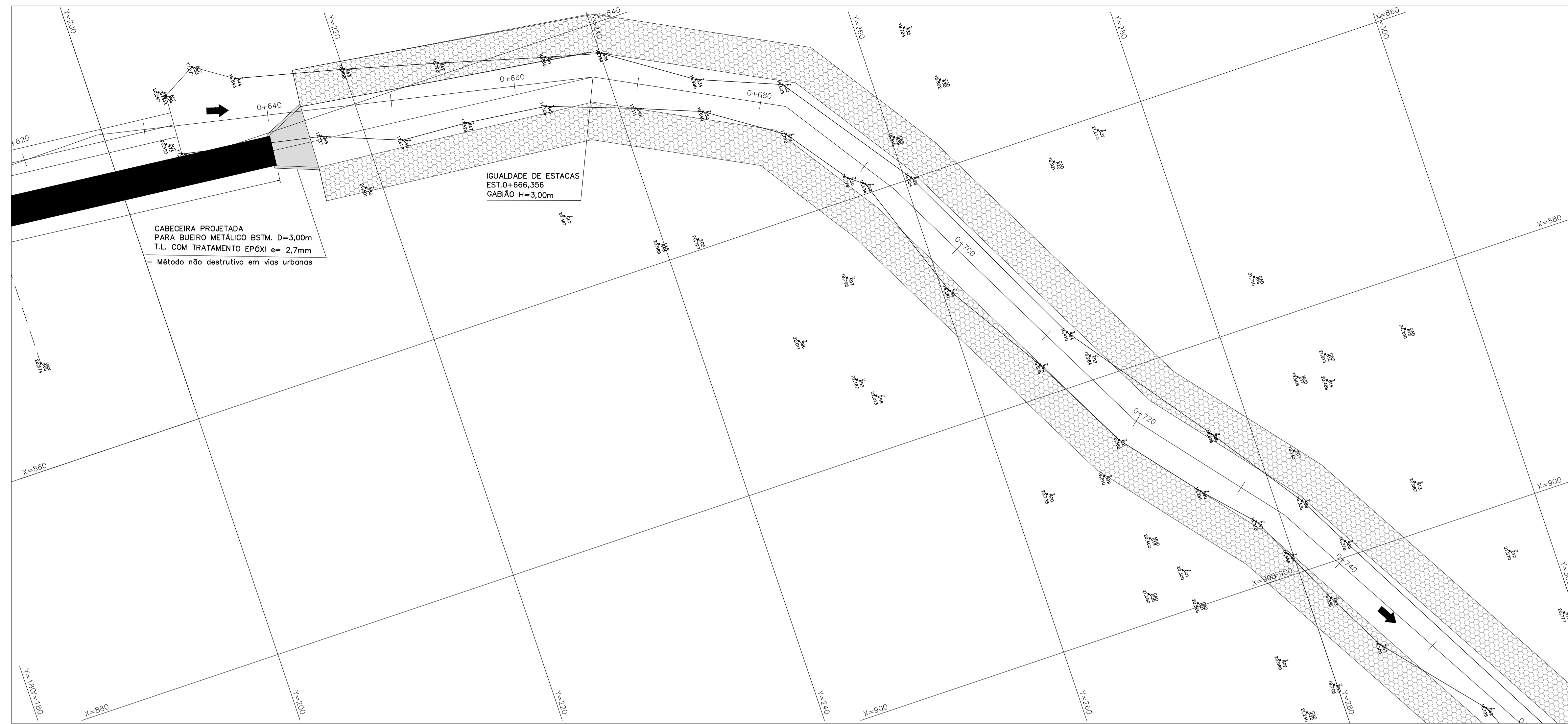
PLANTA BAIXA ESC.: 1:200
