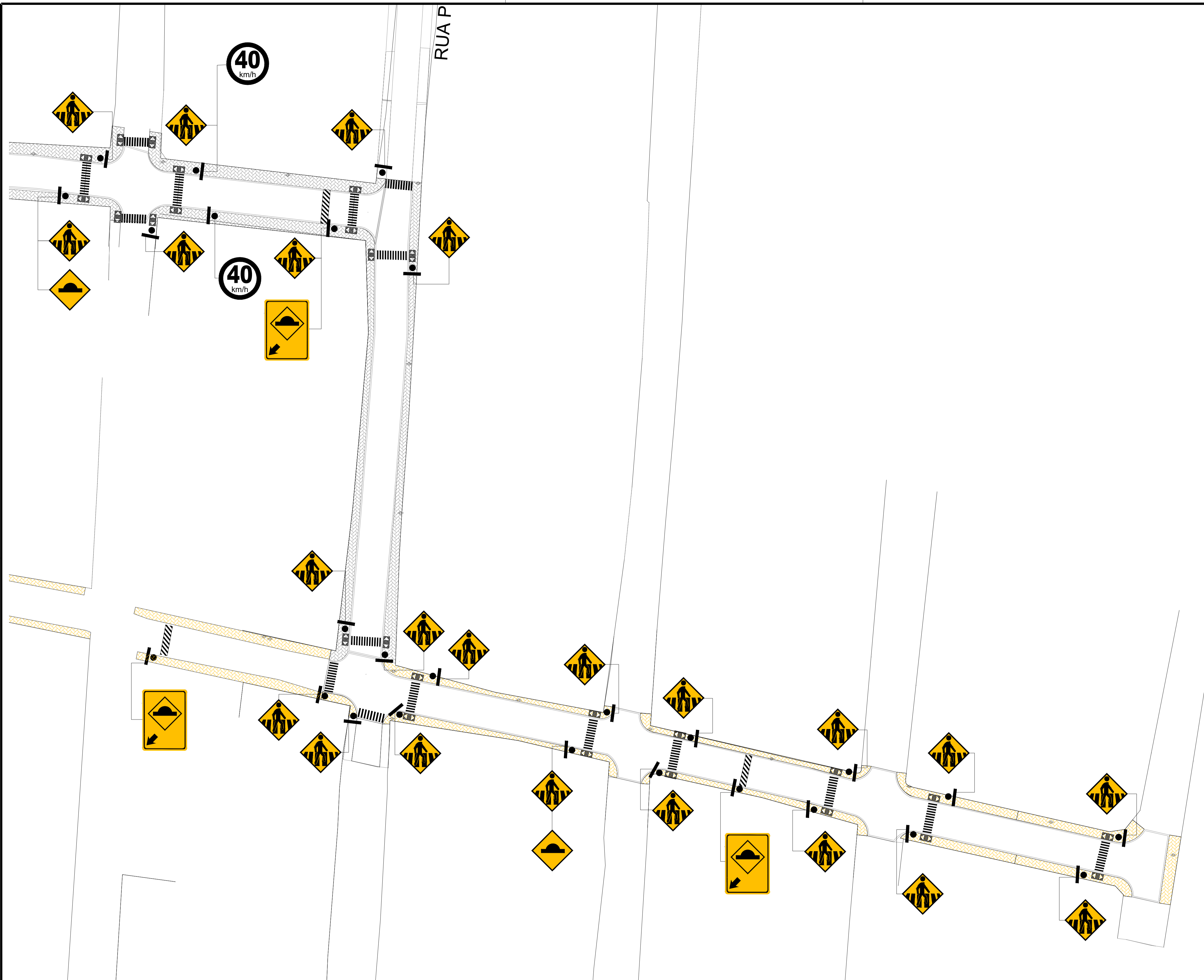
PLANTA BAIXA DE SINALIZAÇÃO ESCALA 1:450
