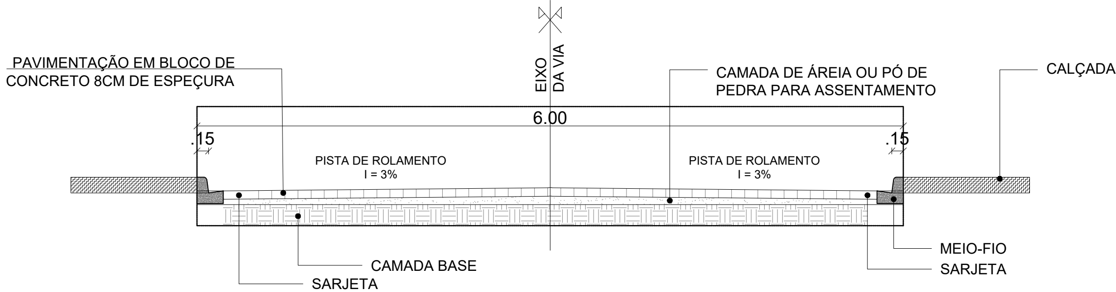
SESSÃO TIPO DA VIA SEM ESCALA
